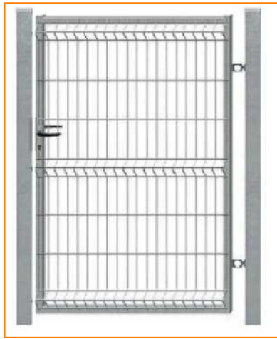
FURTKA OCYNKOWANA 100/2200 Z KLAMKĄ I ZAMKIEM
